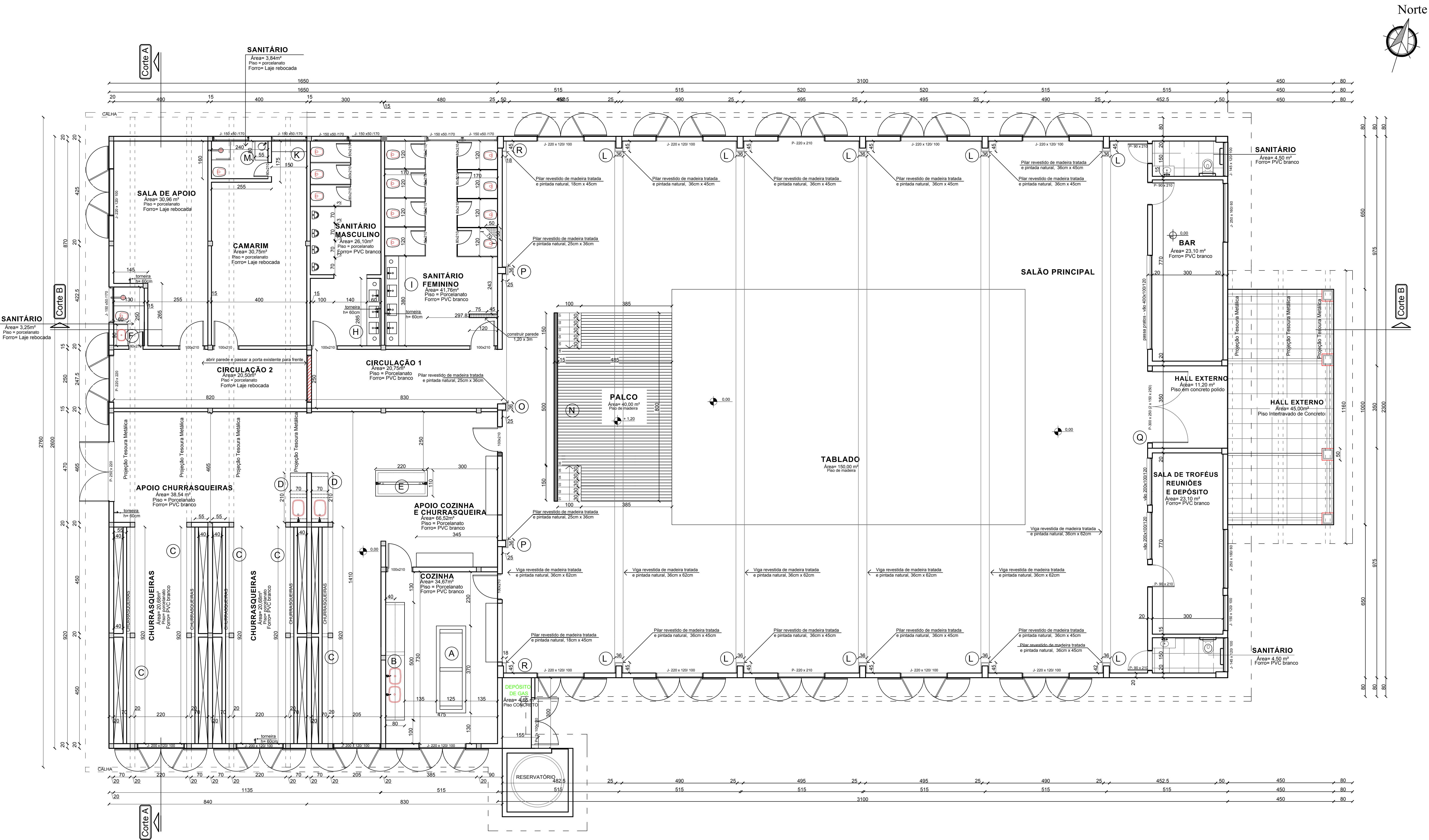
PLANTA BAIXA Escala = 1:75 A = 263,40m2
